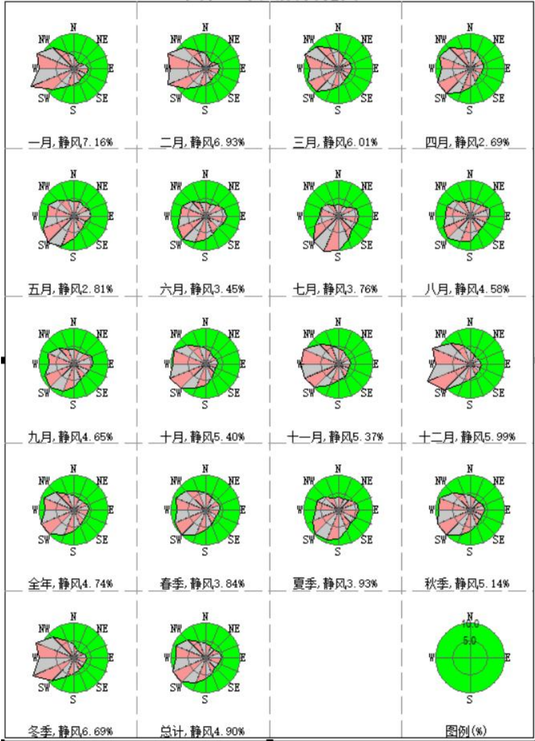
图 5.1-1 肇源气象站（2003-2024 年）各月风向频率玫瑰图 表 5.1-2 肇源气象站（2003-2024 年）各月及年风向风频统计
