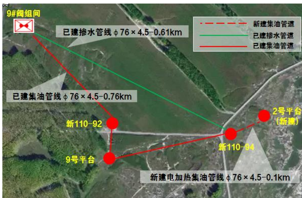
图 3.2-11 挂接新肇联 9#阀组间 3 环电加热管线路由示意图
