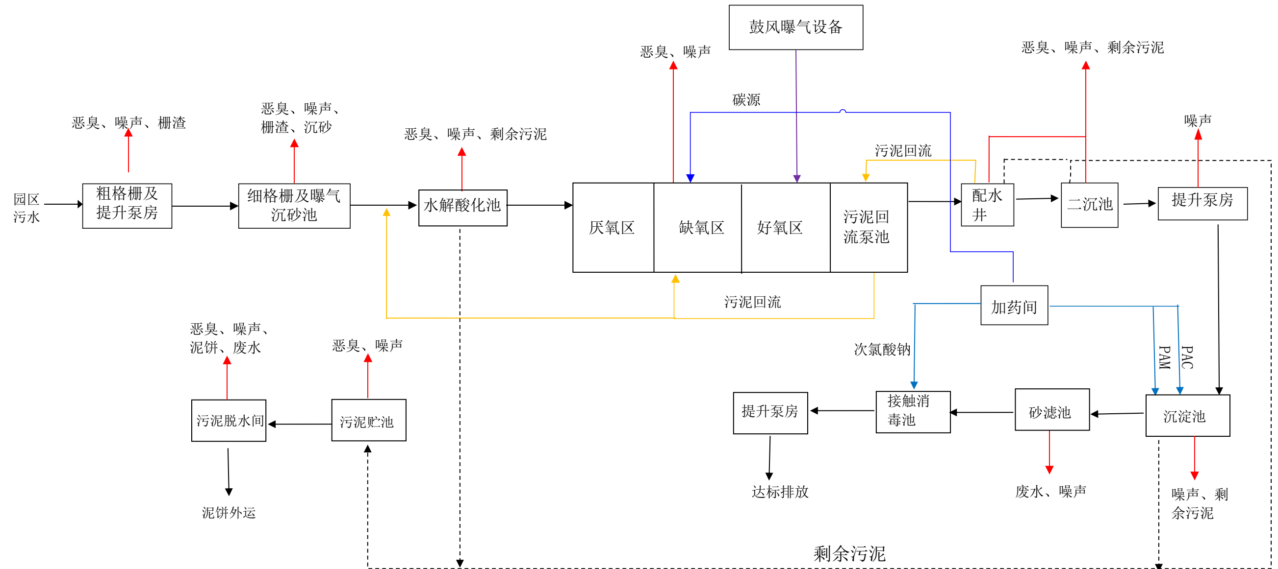
图3.2-1 工程污水处理工艺流程及产污节点图
